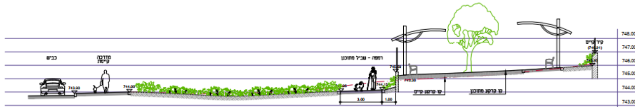
חתך 1-1
