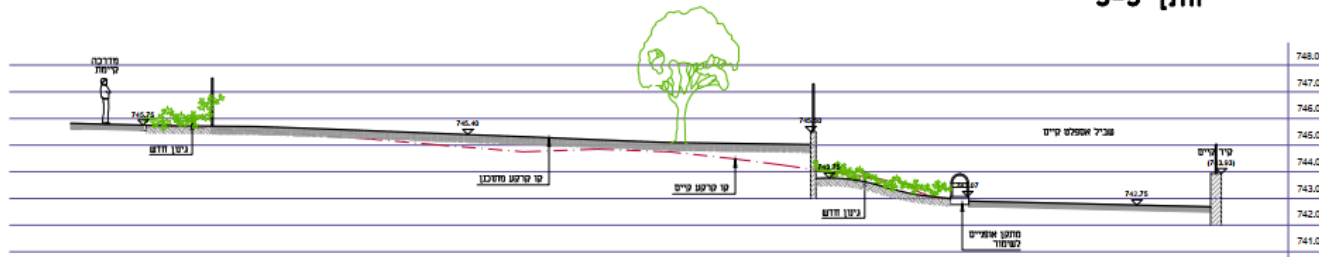
חתך 4-4
