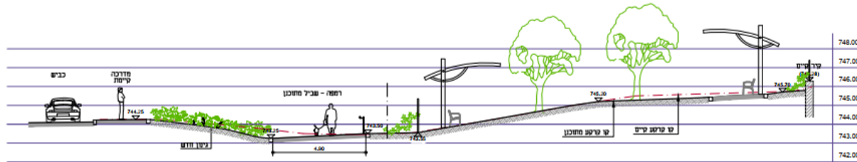
חתך 2-2
