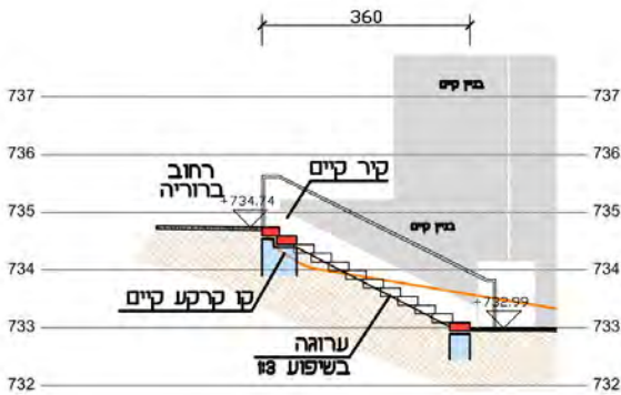
חתך ה-ה
