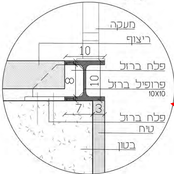
הגדלה חיבור מעקה לרמפה קני"מ 100
