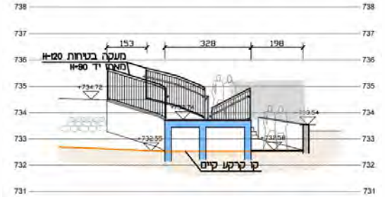
חתך ד-ד
