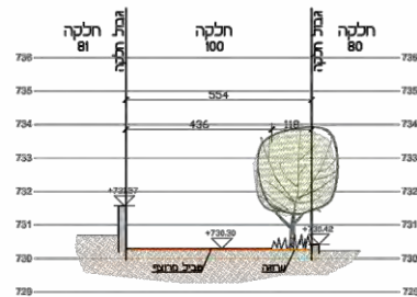
חתך ד-ד
