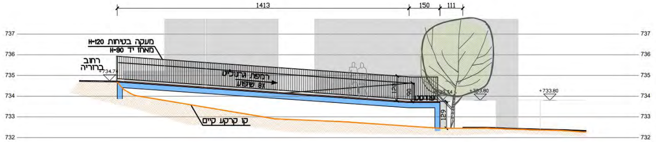
חתך א-א
