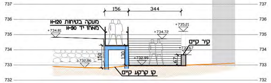
חתך ב-ב
